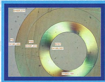
3層 チューブ (内層フッ素樹脂)
