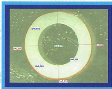
3層 チューブ (外径超薄膜)
