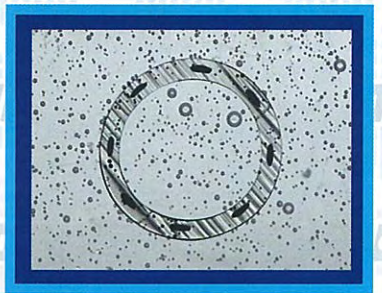
外径0.3mm 中心静脈用フッ素チューブ (造影剤入)
