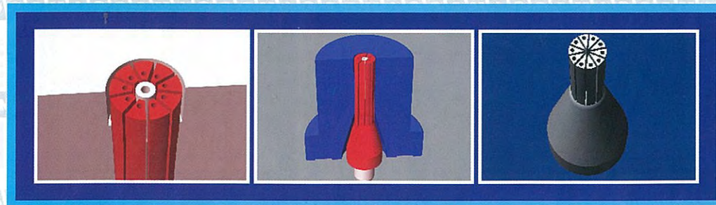
マルチルーメン用ダイの基本概念図 Concept draws of multilumen Head
