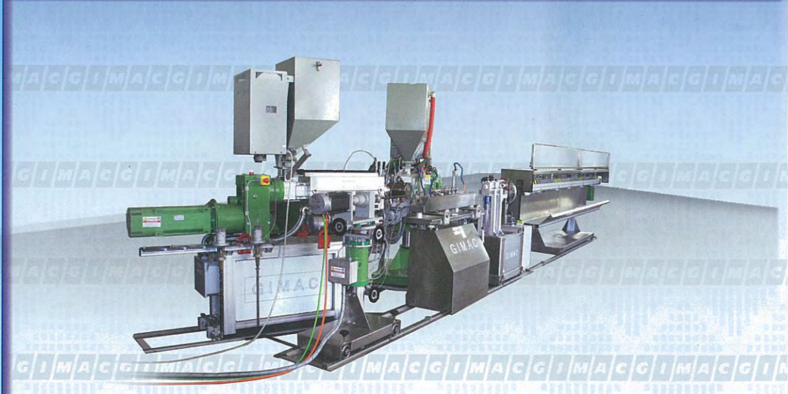
メタルワイヤー入 スパイラルチューブ Metal wire embedded spiral tube
