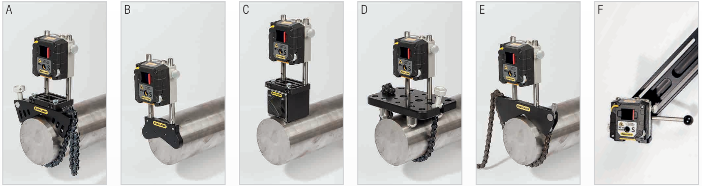
A. オフセットブラケット Part No. 12-1008
